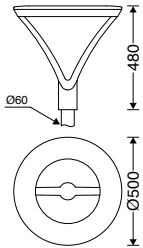
M6094LED...
